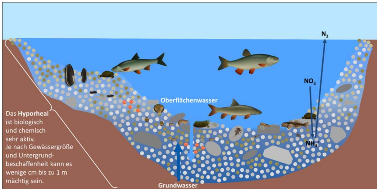
Abbildung 1: Schematische Darstellung des Kieslückensystems (Hyporheal); die wichtigsten Funktionen sind der Austausch zwischen Grund- und Flusswasser, der biochemische Ab- und Umbau von organischen Verbindungen (Selbstreinigung) und die Bereitstellung eines Lebensraums für Wirbellose bzw. Fischeier und -larven.
