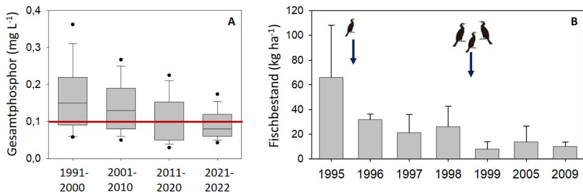
Abbildung 13: Gesamtposphorkonzentration (A) und mittlere Biomasse großwüchsiger Fische (B) an der Nister (Westerwald), dargestellt als Boxpot (Linie: Median, Box 25%-75% der Werte, Punkte: 5%-95% der Werte) und als Balken für Mittelwerte ( \pm Standardabweichung).
